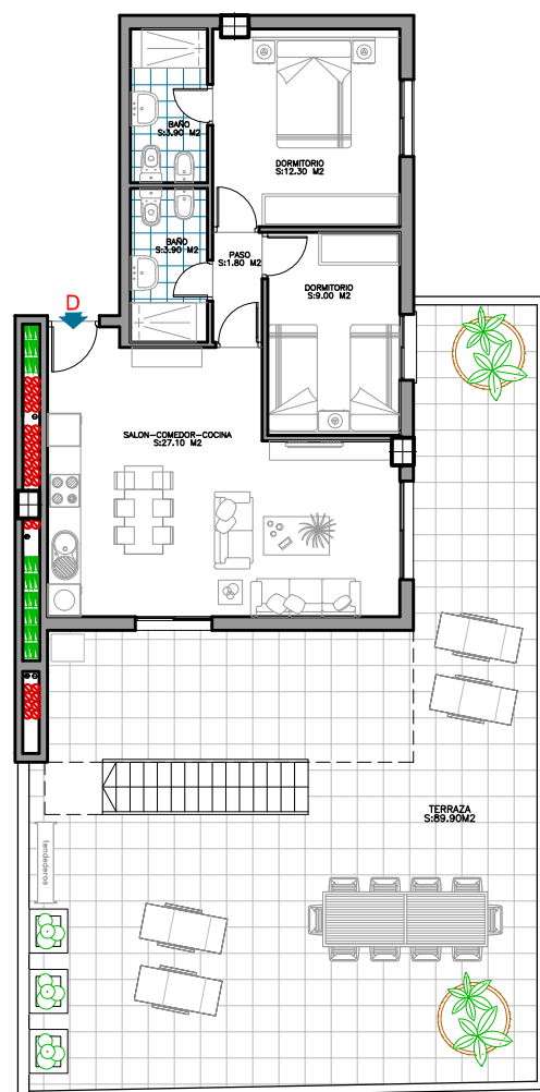
PLANTA ATICO
